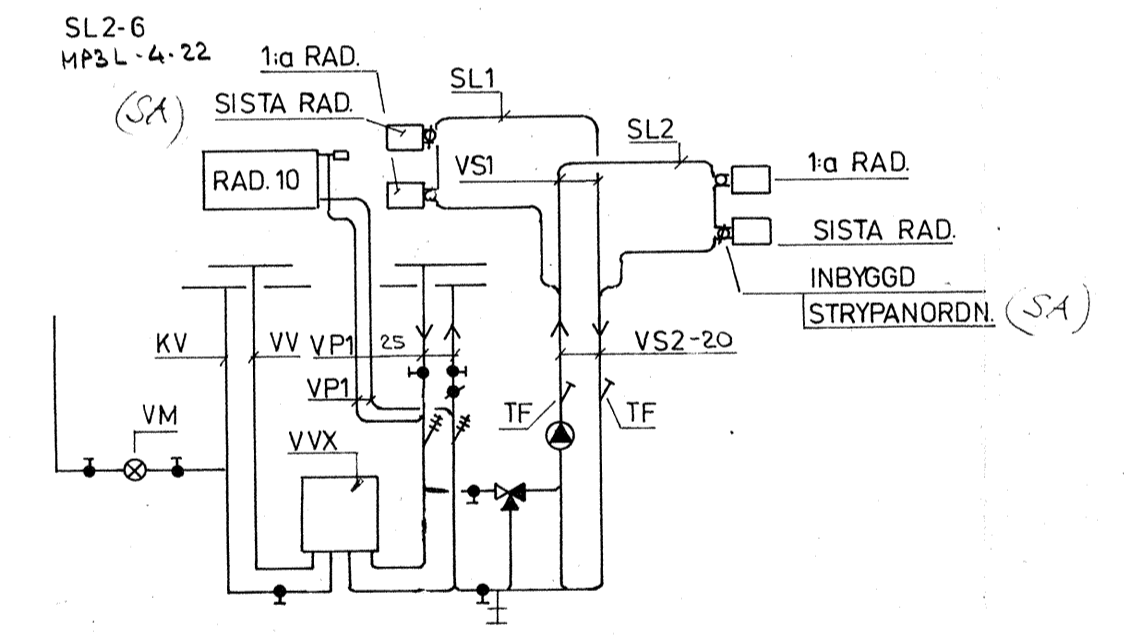
DETALJ INKOPPLING AV VVX
